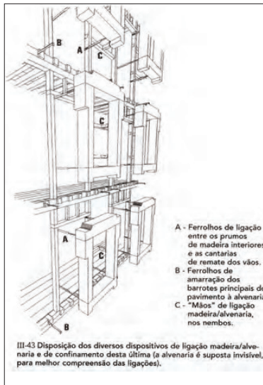
Reabilitação estrutural de edifícios antigos - Vítor Córias. Disposição dos dispositivos de ligação
